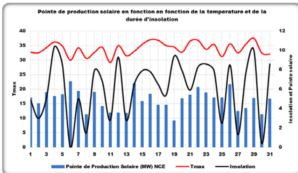
Figure 5 : Evolution de la pointe de production d'énergie solaire en fonction de la température maximale et de la durée d'insolation au cours du mois d'Août 2023.
