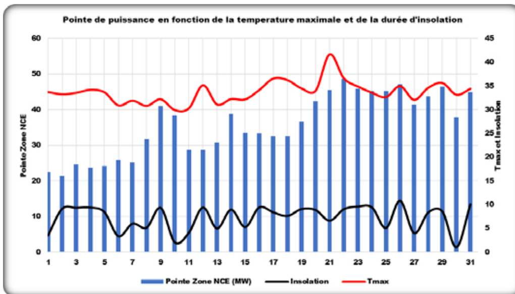
Figure 4 : Evolution de la pointe de puissance en fonction de la température maximale et de la durée d'insolation au cours du mois d'Août 2023
