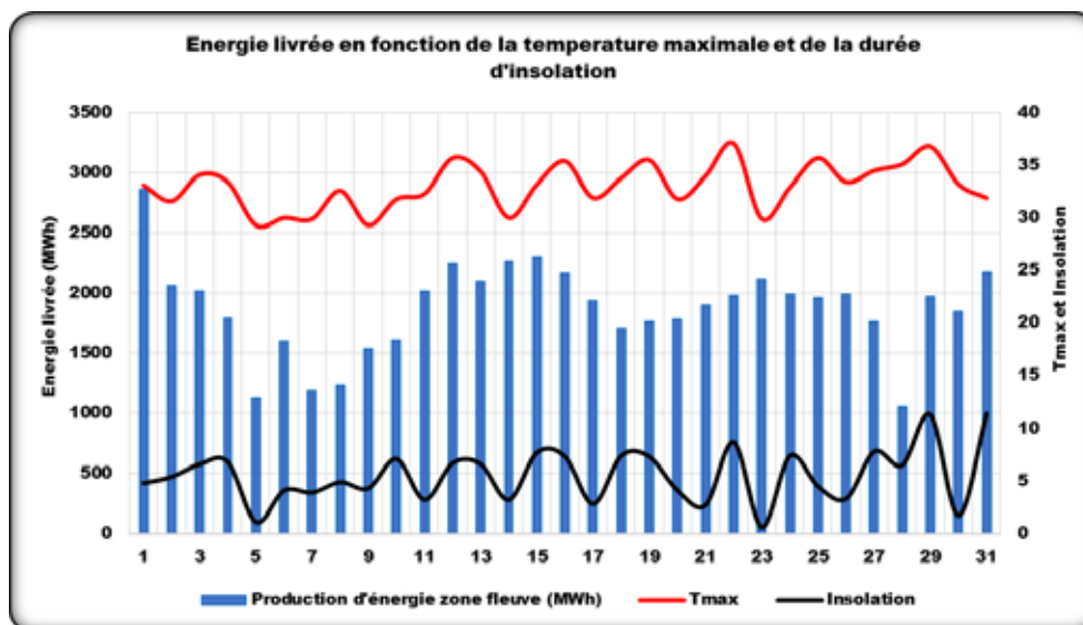
Figure 1 : Evolution de la Quantité d'énergie livrée en fonction de la température maximale et de la durée d'insolation à Niamey au cours du mois d'Août 2023.
