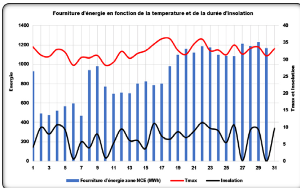
Figure 3 : Evolution de la production d'énergie en fonction de la température maximale et de la durée d'insolation (Zone NCE)
