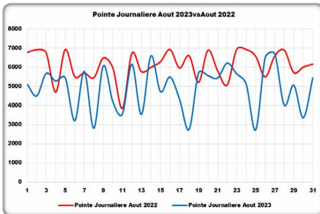
Figure 6 : Comparaison de la pointe de production solaire du mois Août 2023 vs Août 2022.
