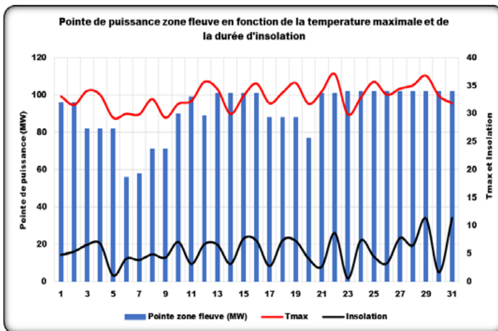
Figure 2 : Evolution de la pointe de puissance par rapport à la température et de la durée d'insolation maximale au cours du mois d'Août 2023
