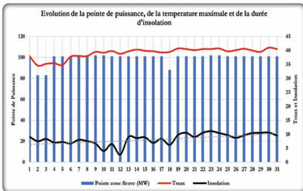
Figure 2 : Evolution de la pointe de puissance, de la température et de la durée d'insolation au cours du mois d'octobre 2023.
