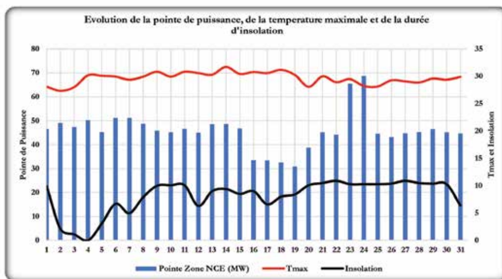
Figure 4 : Evolution de la pointe de puissance, de la température maximale et de la durée d'insolation au cours du mois d'octobre 2023
