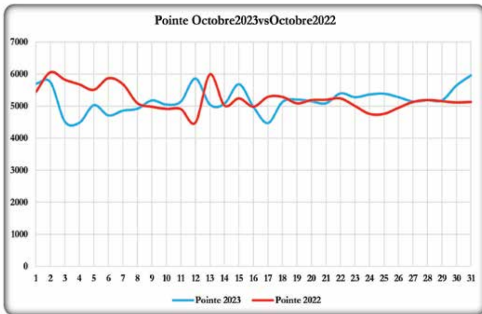
Figure 6 : Analyse de la pointe de production solaire du mois d'octobre 2023 vs octobre 2022 au niveau de la centrale solaire de Malbaza.
