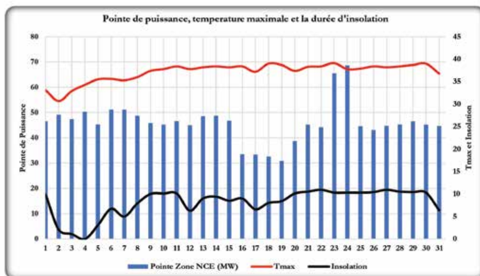
Figure 5 : Evolution de la pointe de production d'énergie solaire, de la température maximale et de la durée d'insolation au niveau de la centrale solaire de Malbaza au cours du mois d'octobre 2023.
