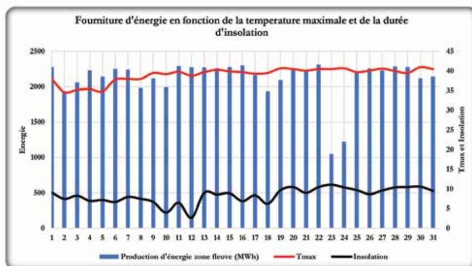
Figure 1 : Evolution de la quantité d'énergie livrée, de la température et de la durée d'insolation au cours du mois d'octobre 2023.
