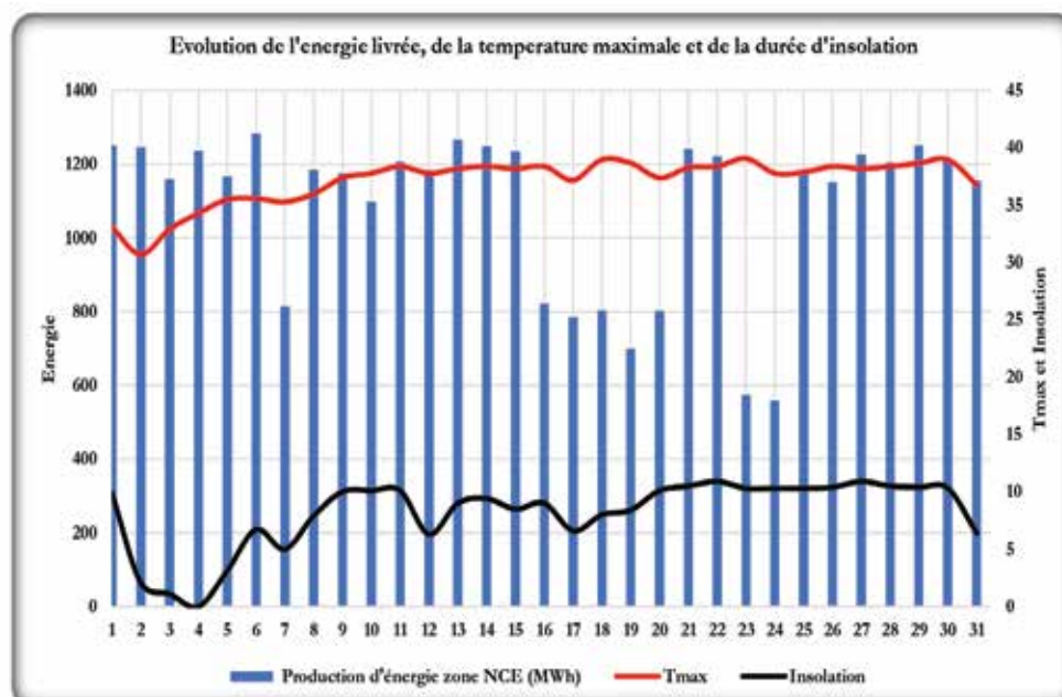
Figure 3 : Evolution de la production d'énergie, de la température maximale et de la durée d'insolation (Zone NCE) au mois d'octobre 2023.
