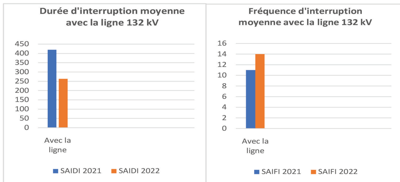
Figure 3 : Variations interannuelles des durées et des fréquences moyennes d'interruption avec la ligne 132 kV (Août 2021-2022).
