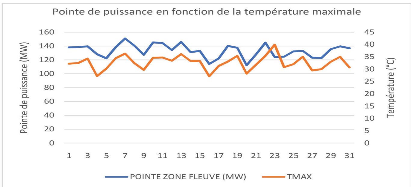
Figure 2 : Evolution de la pointe de puissance par rapport à la température maximale au cours du mois d'août 2022
