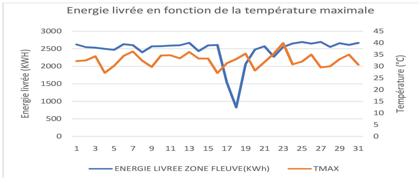
Figure 1 : Evolution de la Quantité d'énergie livrée en fonction de la température maximale dans la zone Fleuve au cours du mois d'Août 2022
