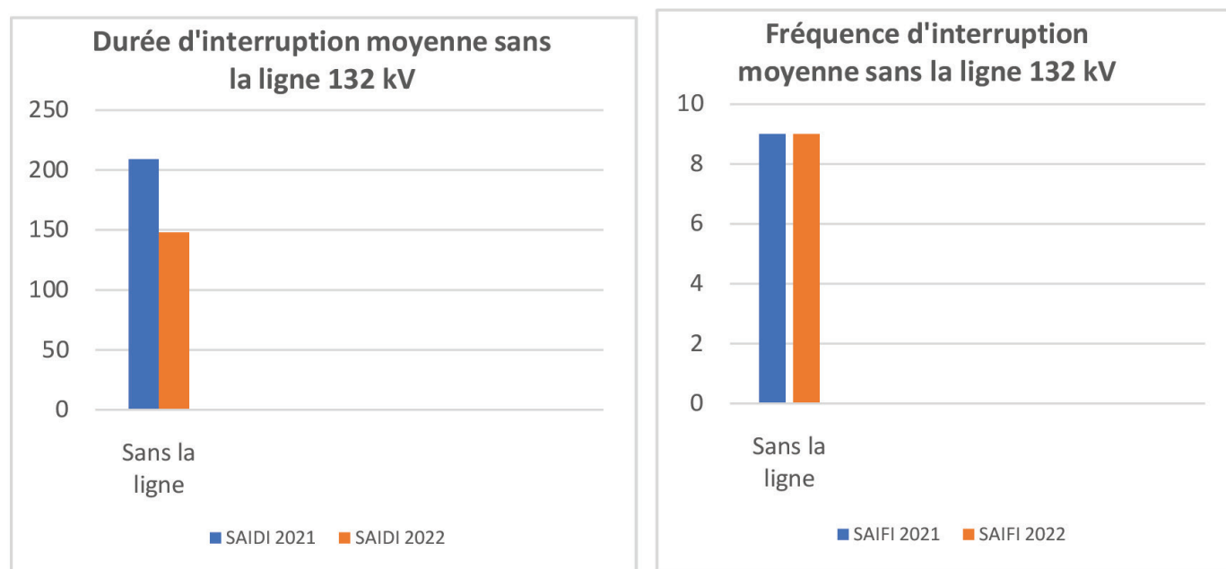
Figure 4 : Variations interannuelles des durées et des fréquences moyennes d'interruption sans la ligne 132 kV (Août 2021-2022).
