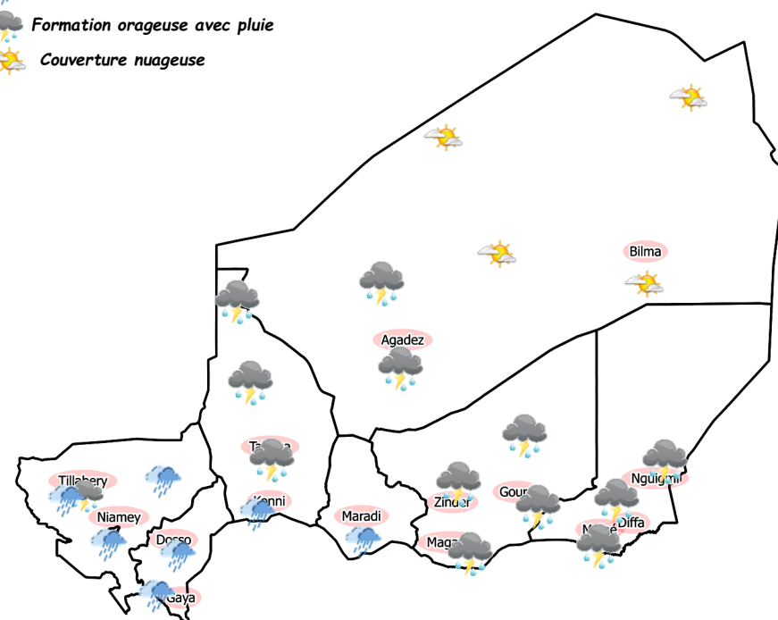
Fig. 1: Temps prévu de la journée du 21 Août 2026
