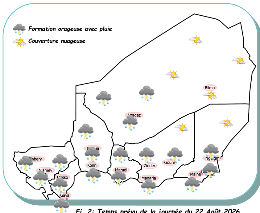
Fi. 2: Temps prévu de la journée du 22 Août 2026
