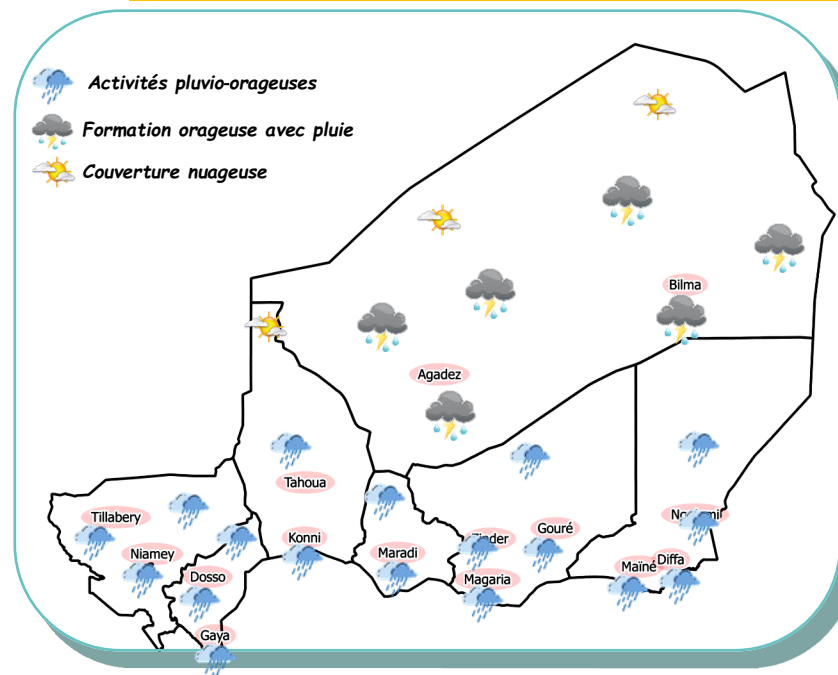
Fig. 3: Temps prévu de la journée du 23 Août 2026
