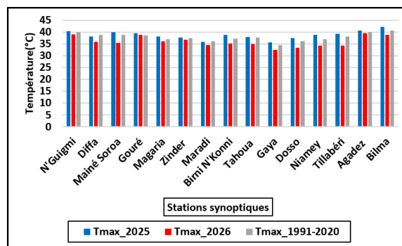
Figure 4: Températures maximales moyennes du 29 septembre au 04 octobre 2026 comparées à la même période de 2025 et à la normale climatologique 1991-2020
